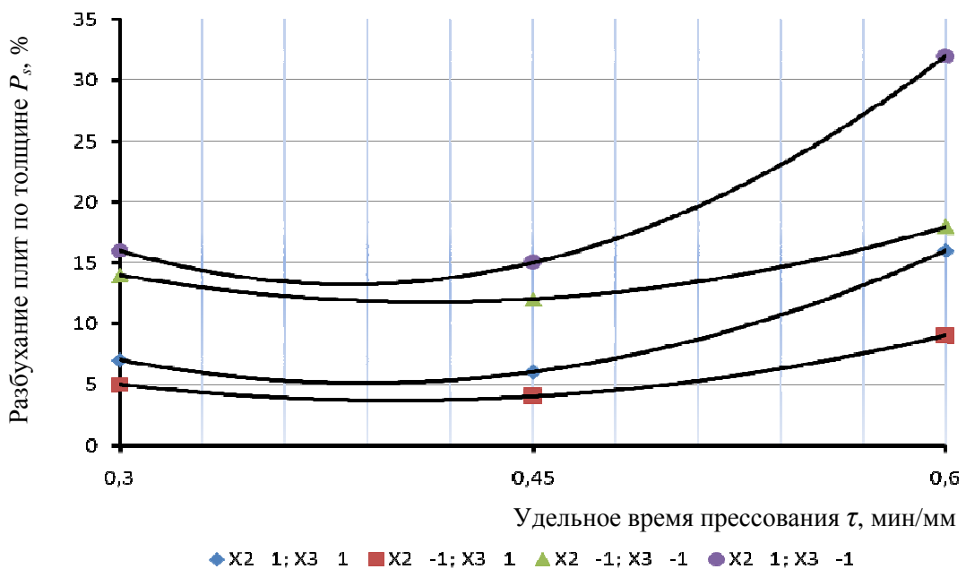
Рис. 5.9. График зависимости разбухания плит по толщине от удельной продолжительности прессования
